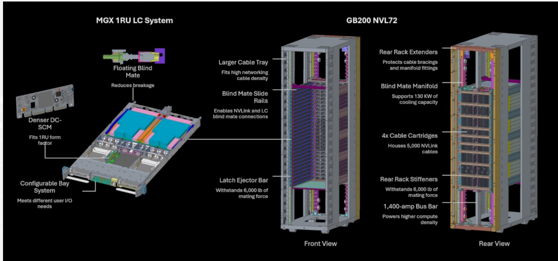
NVIDIA GB200 NVL72 OCP
